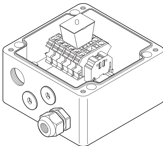
JBU-100-L-E (показан с индикационной лампой)
