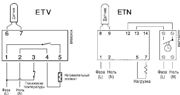
Подключение ETV
